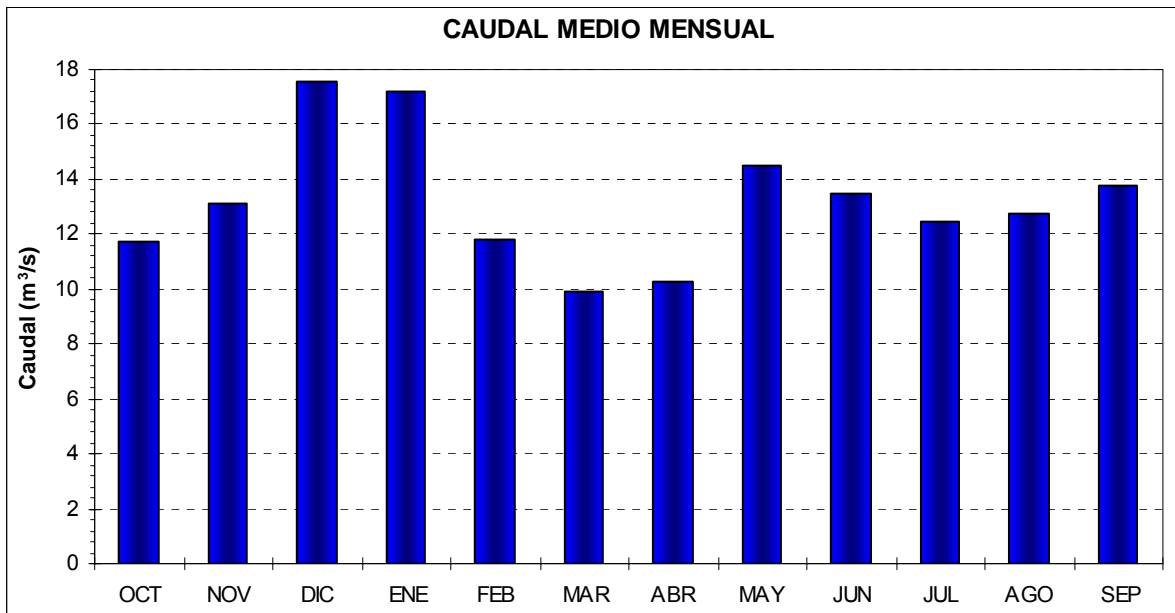
Fig. 1. Régimen Anual del río Alcanadre en el azud localizado en el término municipal de Ontiñena. (Fuente CHE)
