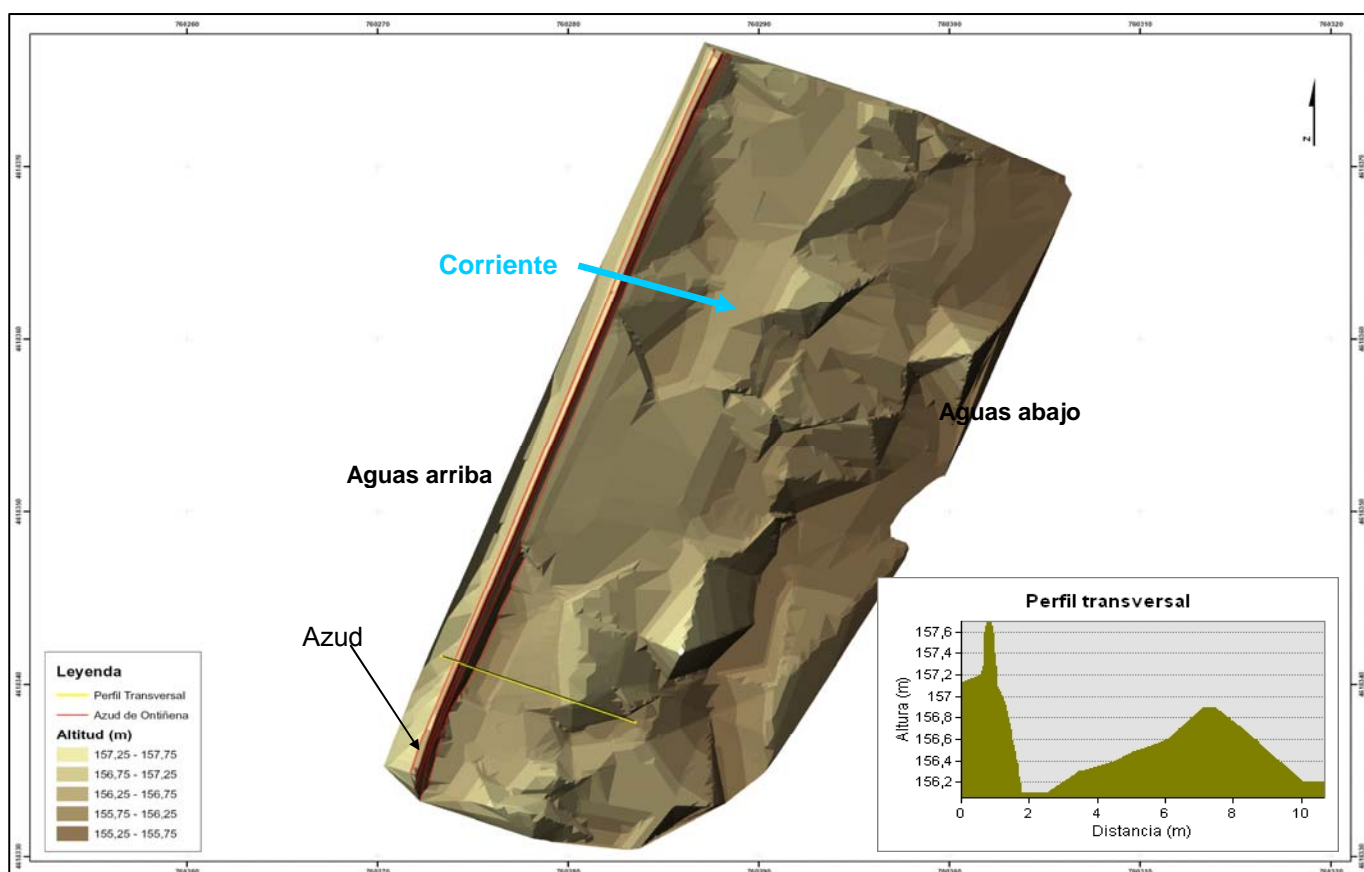
Fig. 6. Modelo Digital de Terreno y Perfil transversal del azud
